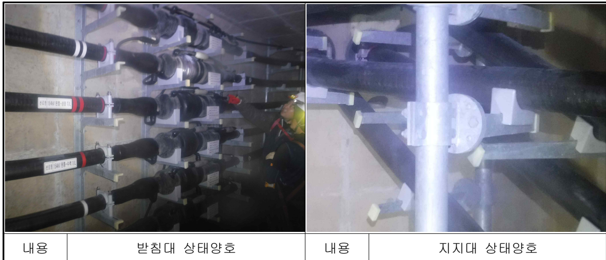
【사진 5.8】 부속 및 부대설비 현황
